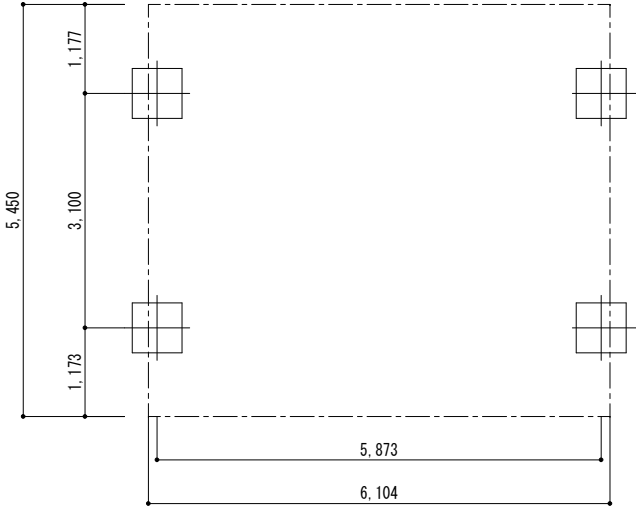
■ 基礎配置図
